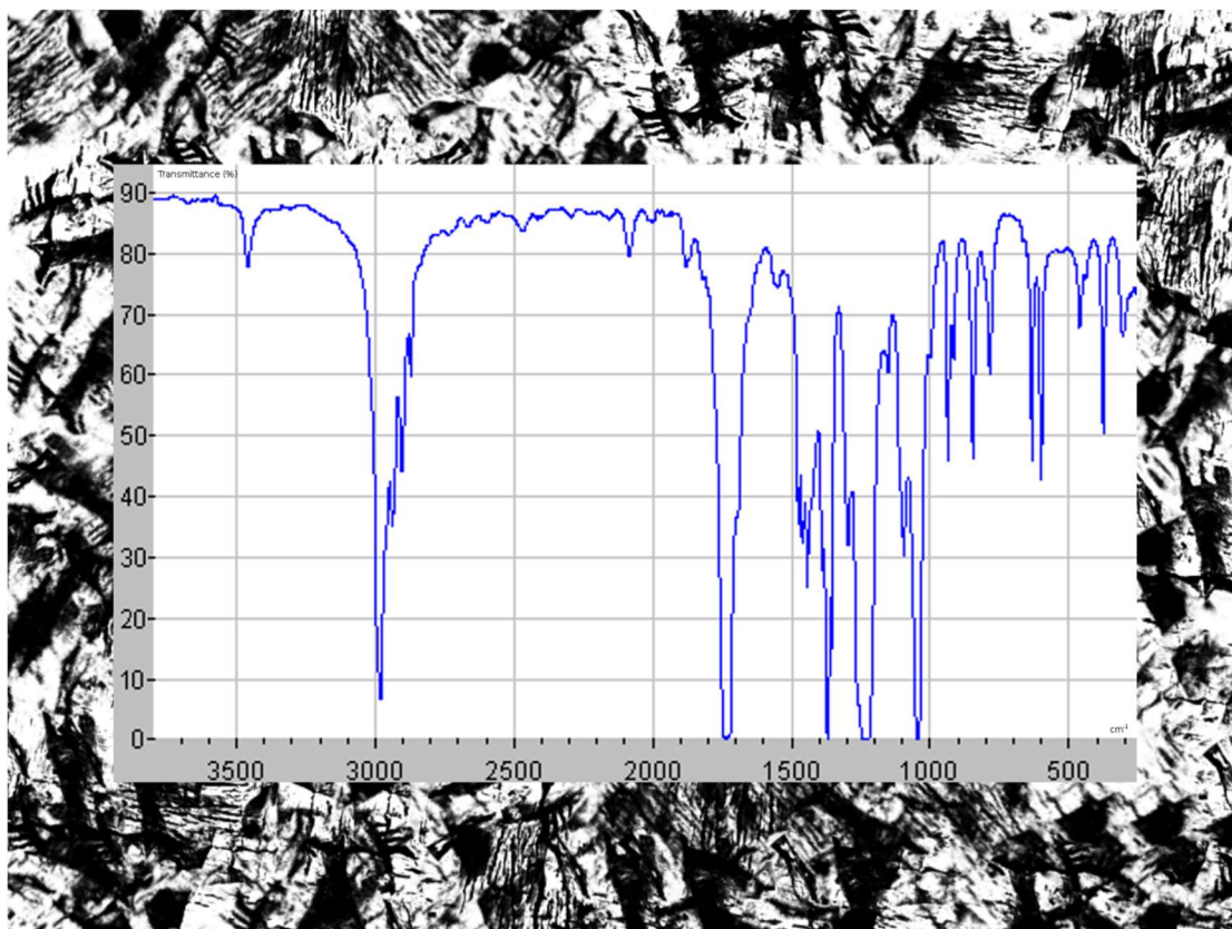
Spectre 2 : C_4H_8O_2
